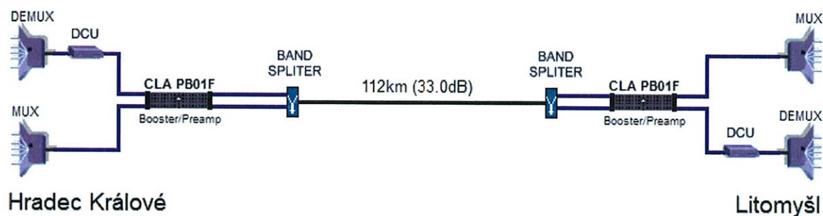
Obrázek 1: Obousměrná jednovláknová DWDM trasa Hradec Králové – Litomyšl
