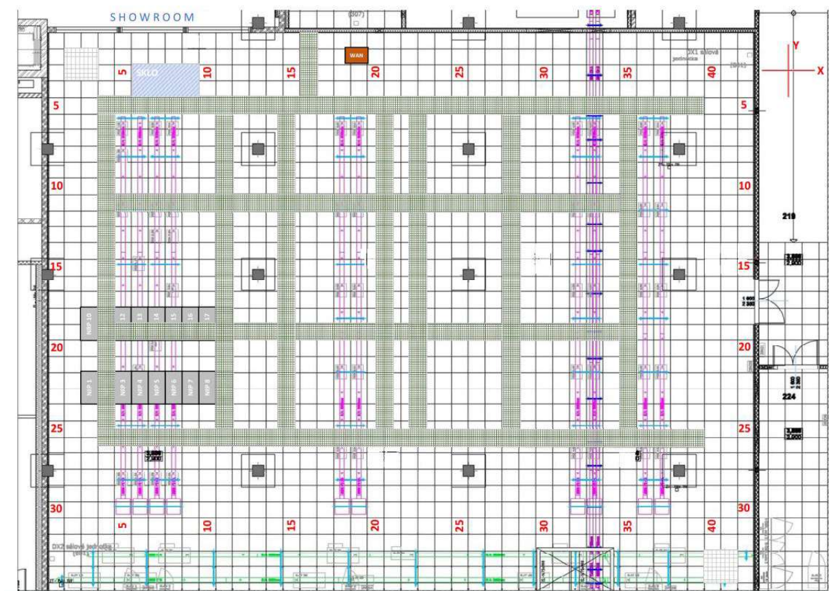
Obr. 2 Kabelové žlaby
