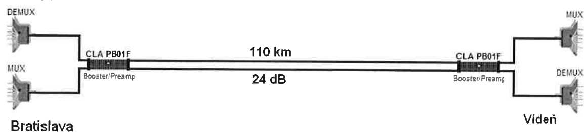
Obrázek 1: Obousměrný dvouvláknový DWDM spoj Bratislava – Vídeň
