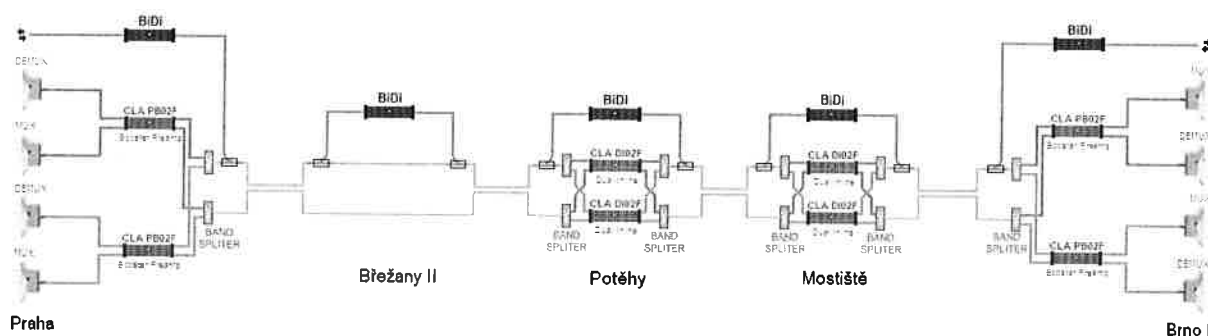
Obrázek 1: Obousměrný kanál vložený do DWDM systému Praha-Brno
