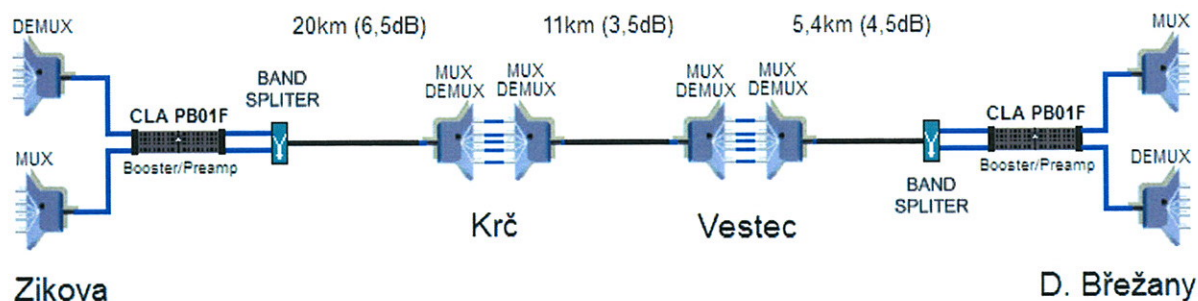
Obrázek 1: Obousměrná jednovláknová DWDM trasa Zikova – Krč – Vestec – Břežany
