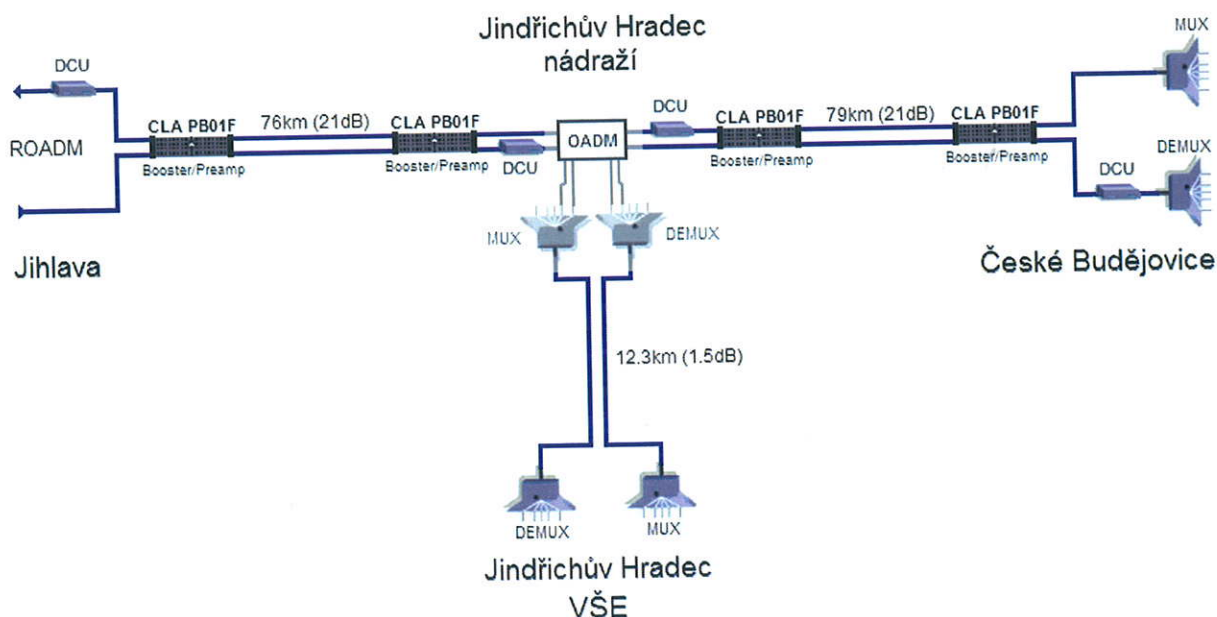
Obrázek 1: Obousměrná dvouvláknová DWDM trasa Jihlava – Jindřichův Hradec – České Budějovice
