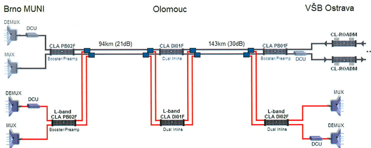
Obrázek 1: Rozšíření obousměrné dvouvláknové DWDM trasy Brno – Olomouc – Ostrava o přenos v L pásmu
