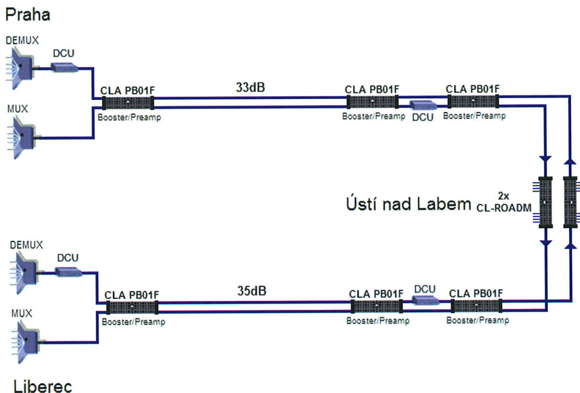
Obrázek 1: Obousměrná dvouvláknová DWDM trasa Praha – Ústí nad Labem – Liberec
