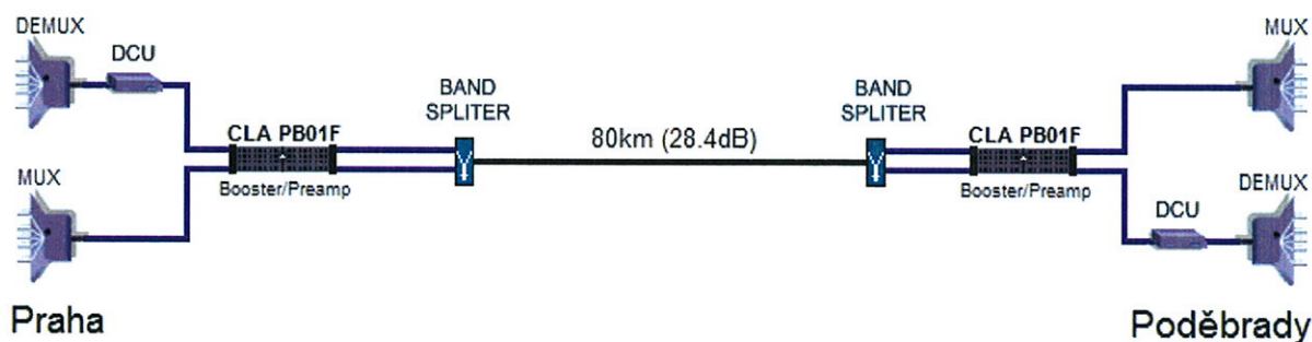
Obrázek 1: Obousměrná jednovláknová DWDM trasa Praha – Poděbrady
